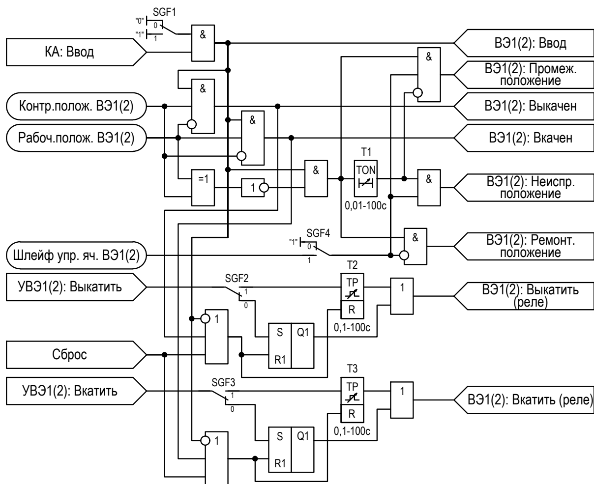
Рисунок 2.59 – Функциональная схема «ВЭ1(2)»
