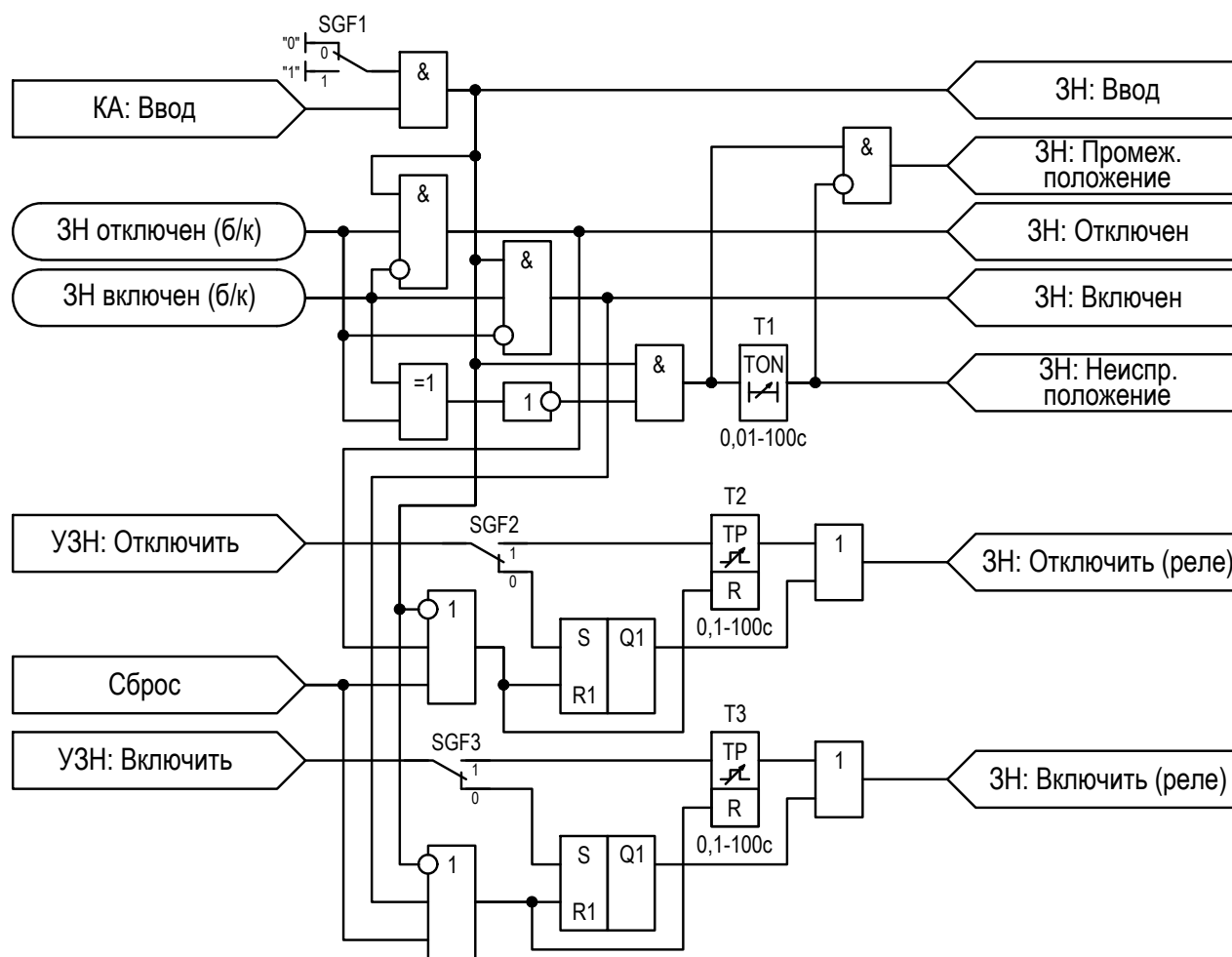
Рисунок 2.58 – Функциональная схема «ЗН»
